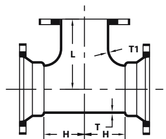
MJ x BRIDA DMF
