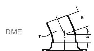
MJ x PE 22 1/2°
