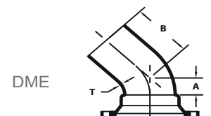
MJ x PE 45°
